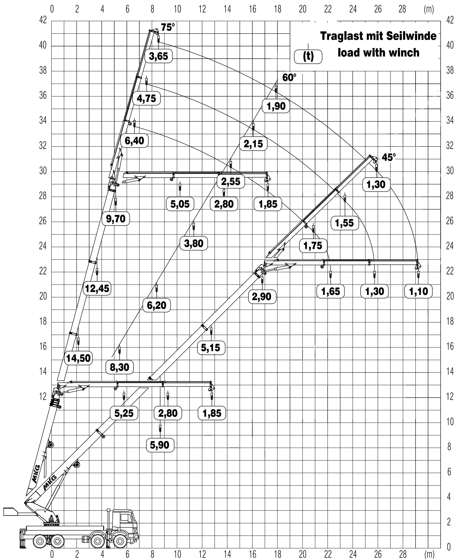
Traglastdiagramm load diagram
